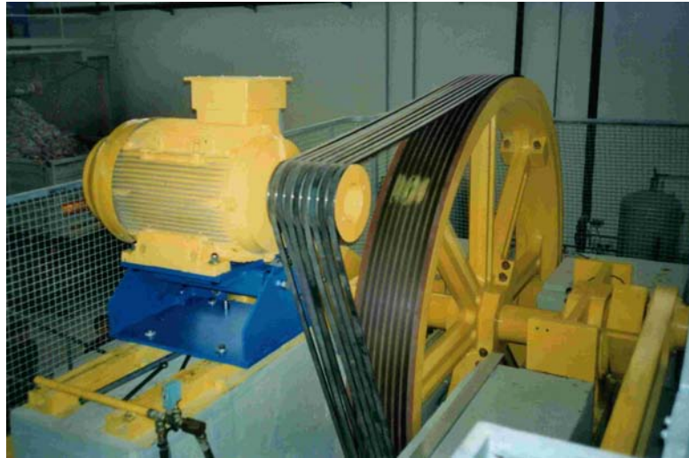
Base de motor en transmisión de depuradora
