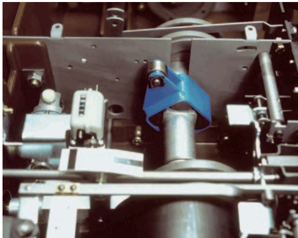
Leva de paso para contadora
