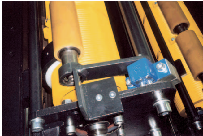
Rodillo prisionero en imprenta
