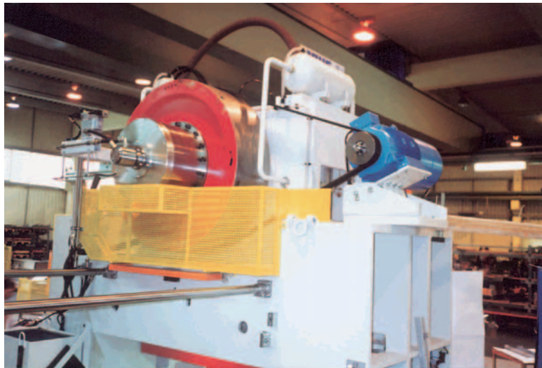
Base de motor en molino de prensa
