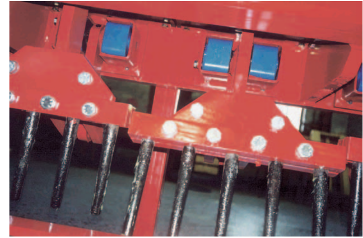
Rastrillo en máquina cosechadora
