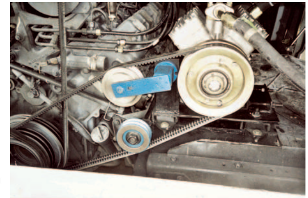
Tensión de correas en compresores A.A de autobuses y autocares
