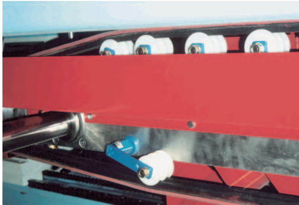
Rodillo de ajuste de correas en maquinaria de evase/embalaje
